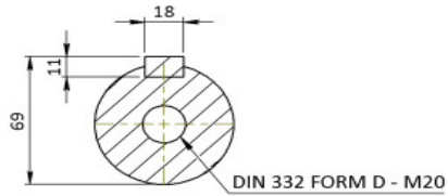
KESİT A-A
